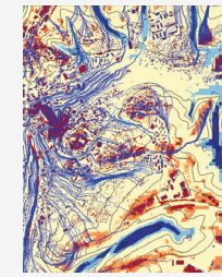
Kaltluftsimulationen
