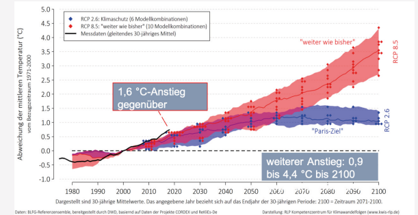
Klimaanalysen
